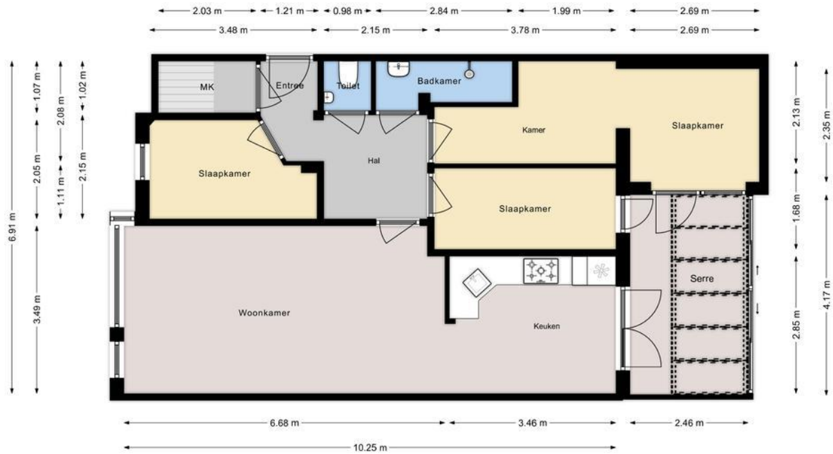
VLIERBOOMSTRAAT 307 Begane grond Hoogte 2.66m
